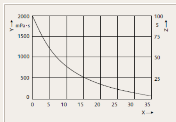
Viscosité d'ACRIFIX® 2R 0190
